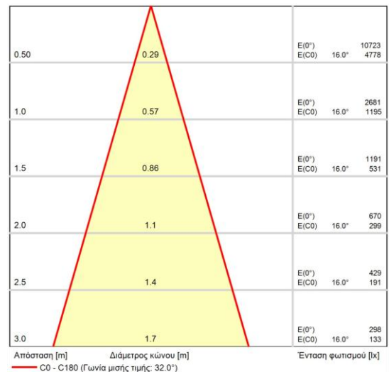
Κωνικό διάγραμμα για Έξοδοι φωτός 1 και 2
