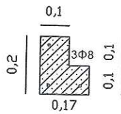
ΕΠΙΣΤΕΨΗ
