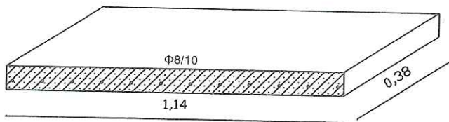
ΠΛΑΚΑ ΣΦΡΑΓΙΣΗΣ
