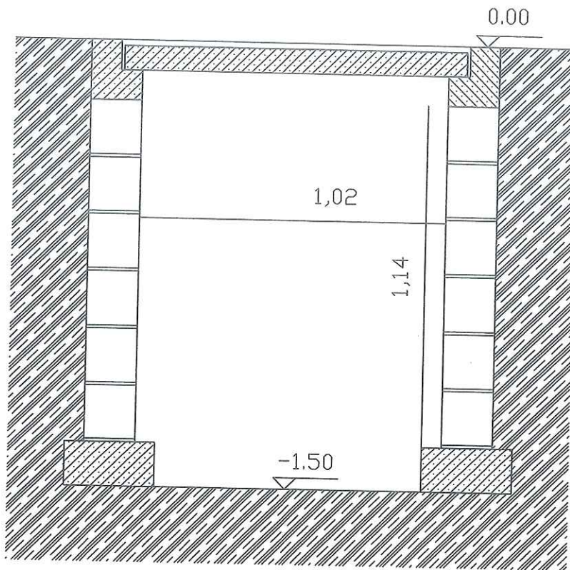
ΤΟΜΗ ΚΛ: 1/20
