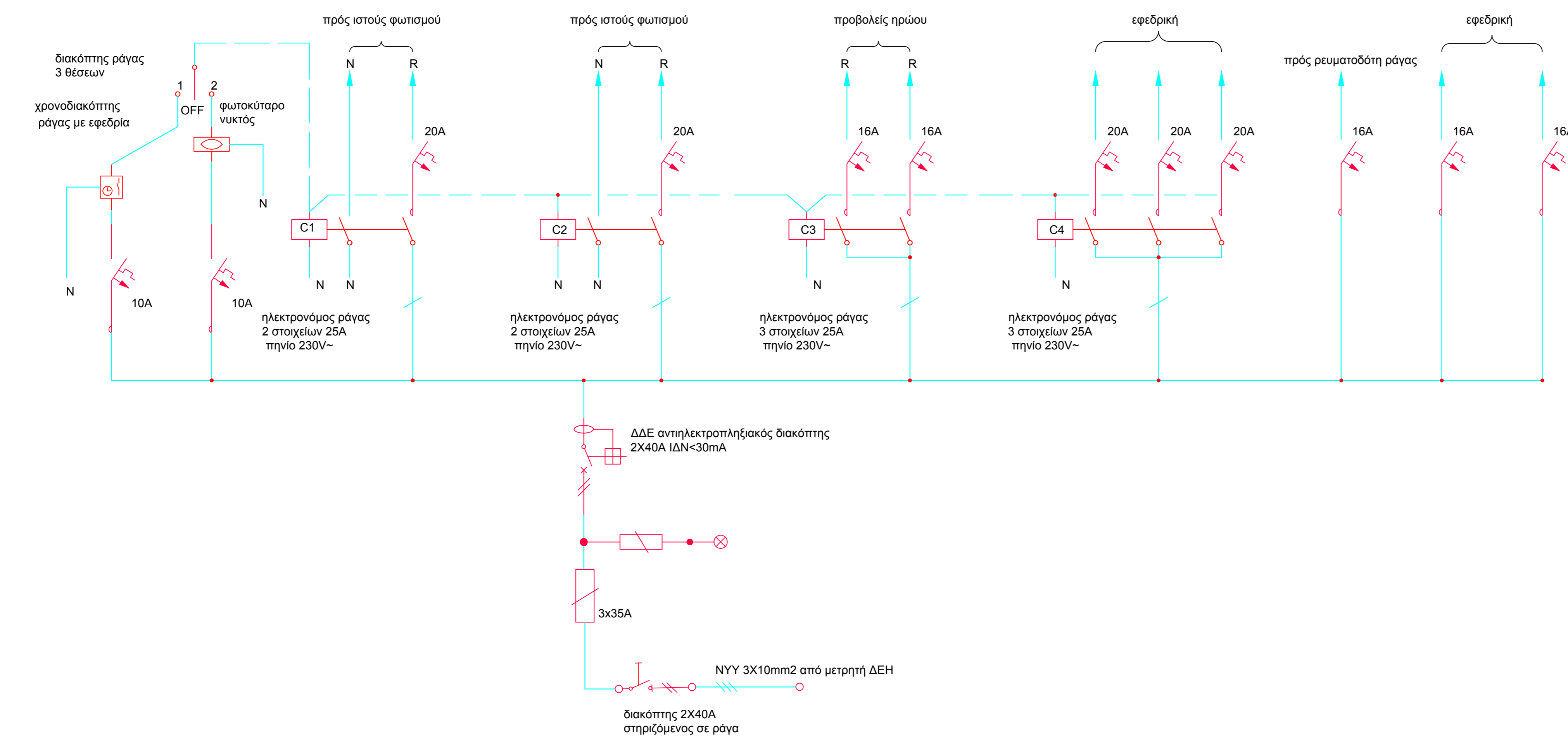
ΗΛΕΚΤΡΙΚΟΣ ΠΙΝΑΚΑΣ ΔΙΑΝΟΜΗΣ
